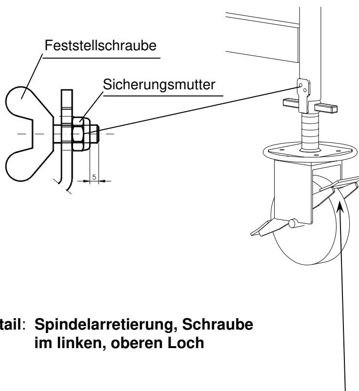
Bild 1: Fahrwerk mit Teleskop-Fahrbalken L228
