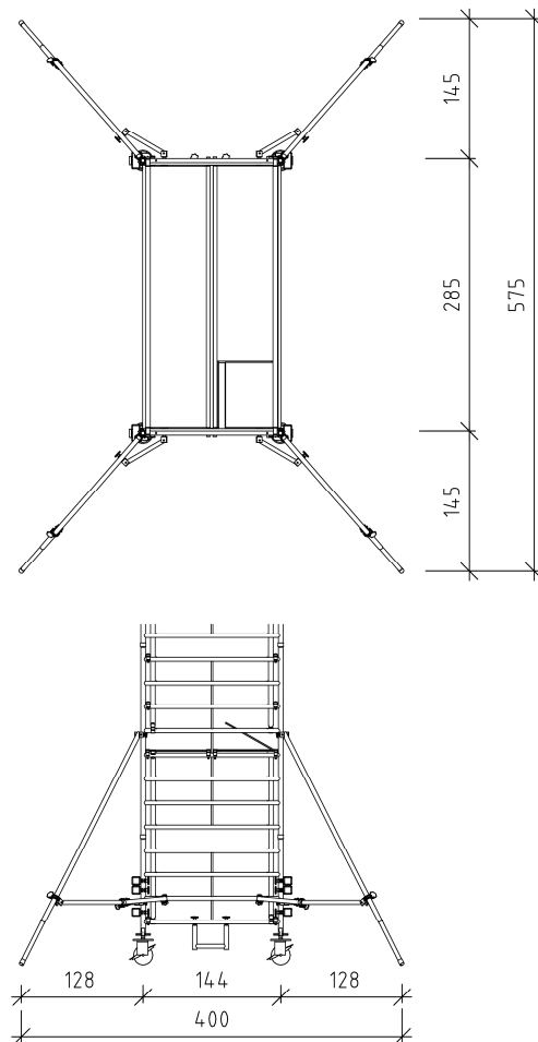
Bild 20: wandseitiger Aufbau
