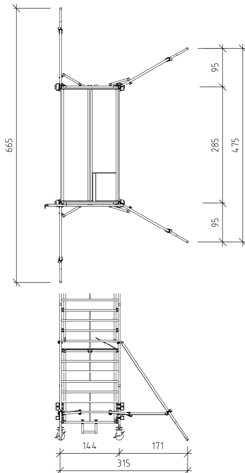
Bild 19: mittiger Aufbau
