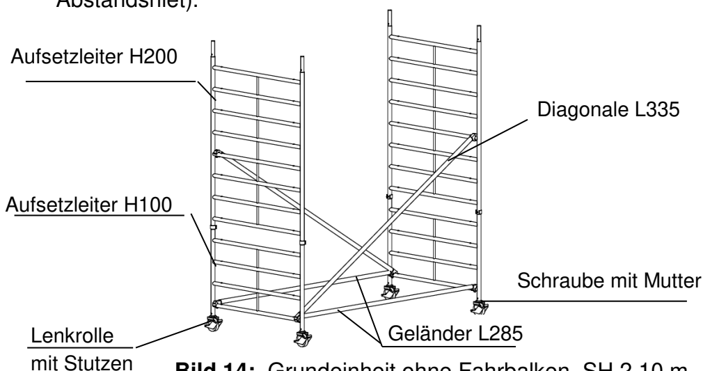
Bild 14: Grundeinheit ohne Fahrbalken, SH 2.10 m
