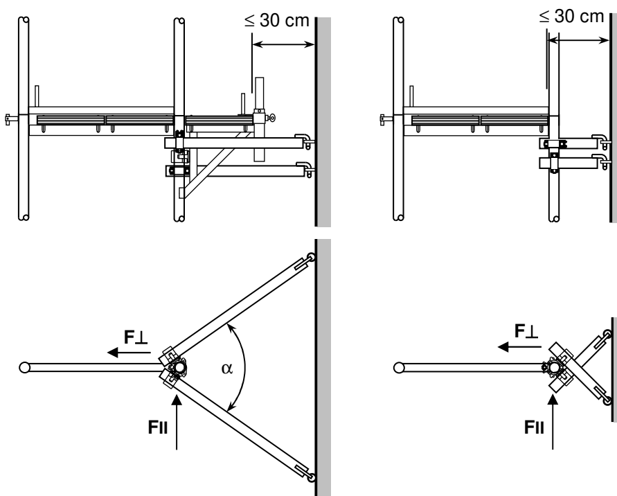
Bild 19: Höhenlage der Dreieckhalter bei Anschluss im „Knoten“
