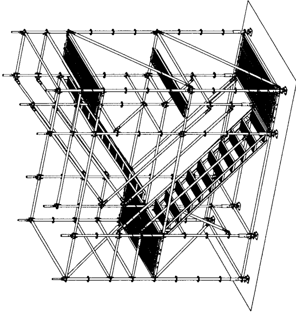
Abbildung 2.1.16: Kompletlierter Seitenschutz in der Mittelage
