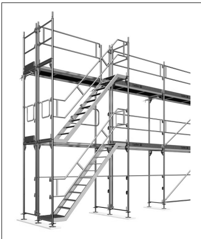
Bild 13: gleichlaufender Treppenaufstieg
