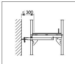
Bild 40: Blitzanker
