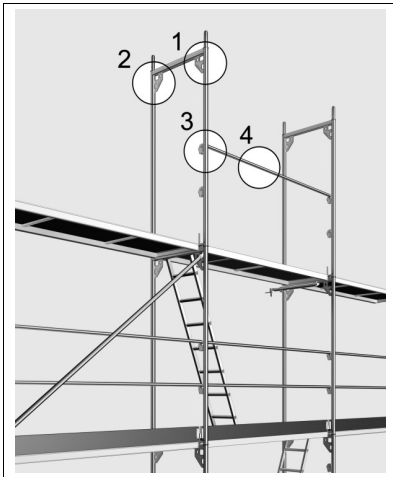
Bild 17: Anschlagpunkte 1, 2, 3 und 4 für PSaGA (Details siehe Bilder 18, 19 und 20)
