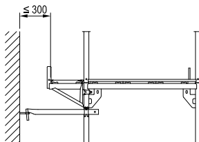
Mit zwei Knotenblechkupplungen in den Knotenblechen angeschlossen.
