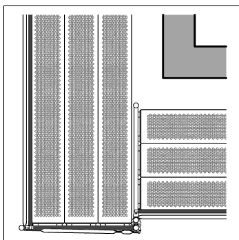
Bild 12: Eckausbildung (Draufsicht)
