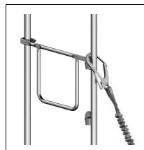
Bild 24-2: Detail Anschlagpunkt 6 Doppelstirngeländer am Geländerkästchen
