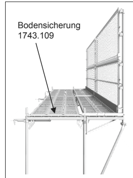
Bild 57: Schutzwand auf Konsole
