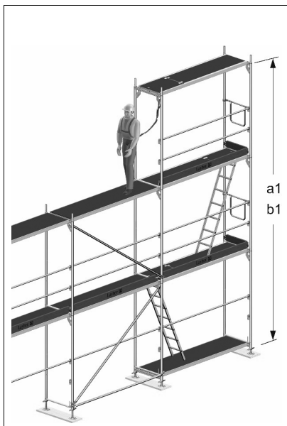
Bild 25: Anschlag über Kopf
