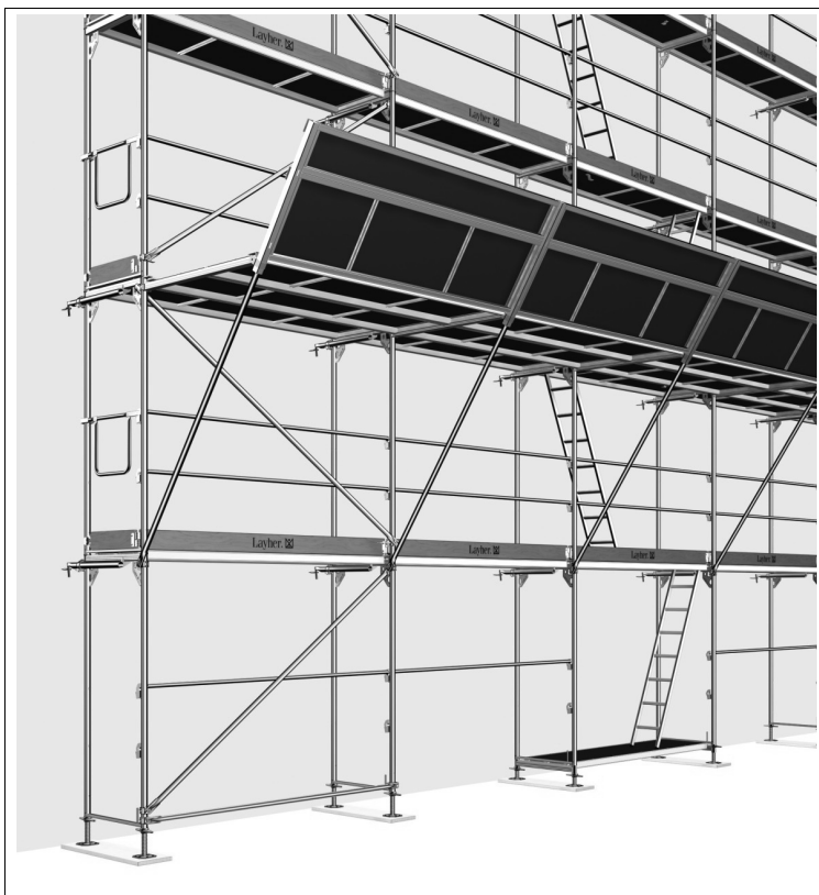
Bild 50: Schutzdach
