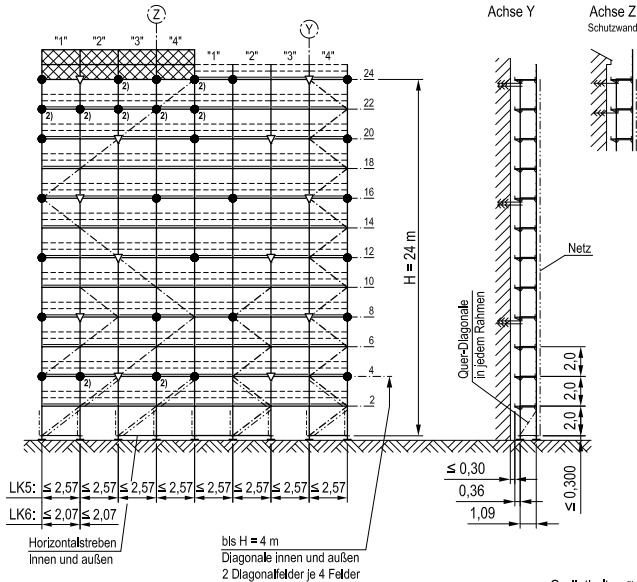
Ankerkräfte [kN]
