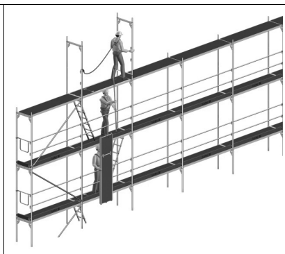
Bild 35: 2. Stellrahmen
