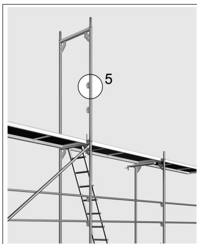
Bild 21: Anschlagpunkt 5 für PSaGA (Detail siehe Bild 23)
