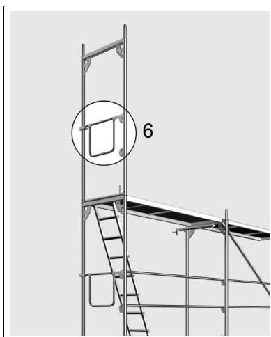
Bild 22: Anschlagpunkte 6 für PSaGA (Detail siehe Bilder 24-1; 24-2)
