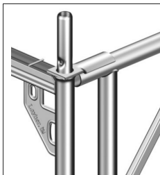
Bild 48: Gitterträger-Endlaschen
