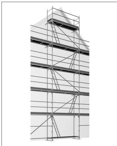
Bild 15: Innen liegender Leitergang
