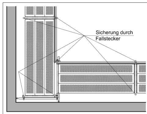
Bild 45: Innen liegende Ecken
