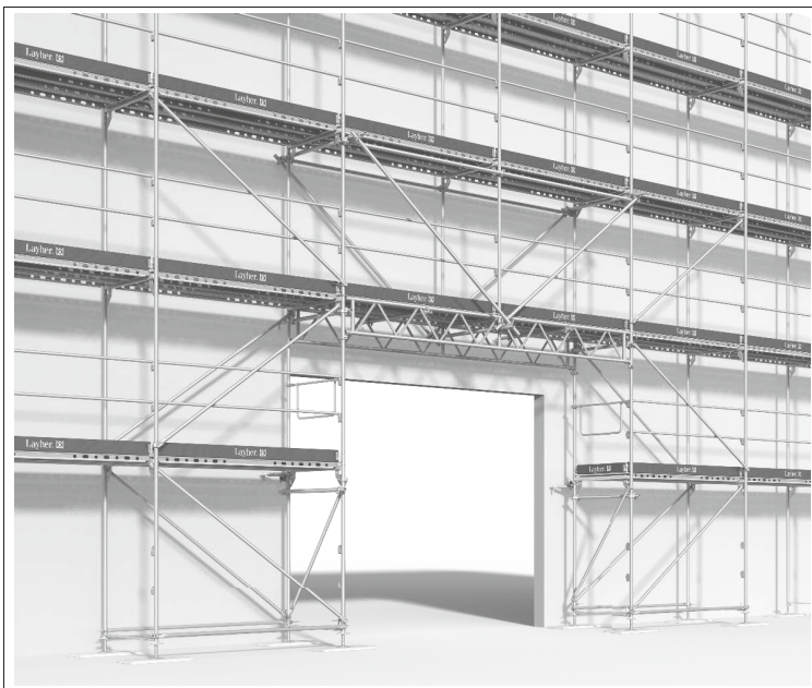
Bild 47: Überbrückung
