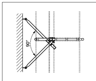
Bild 42: V-förmig angeordnetes Ankerpaar
