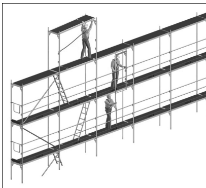
Bild 36: Geländerholm und Böden
