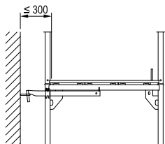
Gerüsthalter "lang" Mit zwei Normkupplungen am inneren und äusseren Ständer angeschlossen.
