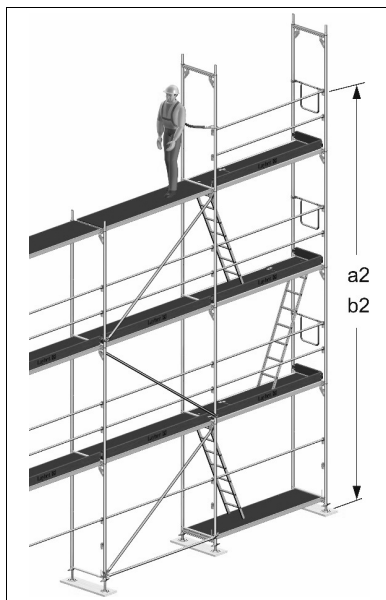
Bild 26: Anschlag auf Geländerholmhöhe
