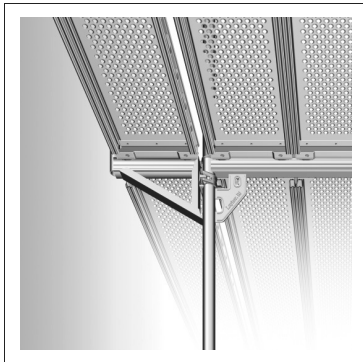
Bild 51: Konsole 0,36 m
