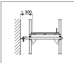
Bild 39: Gerüsthalter „lang“
