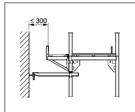
Bild 41: Gerüsthalter „kurz“
