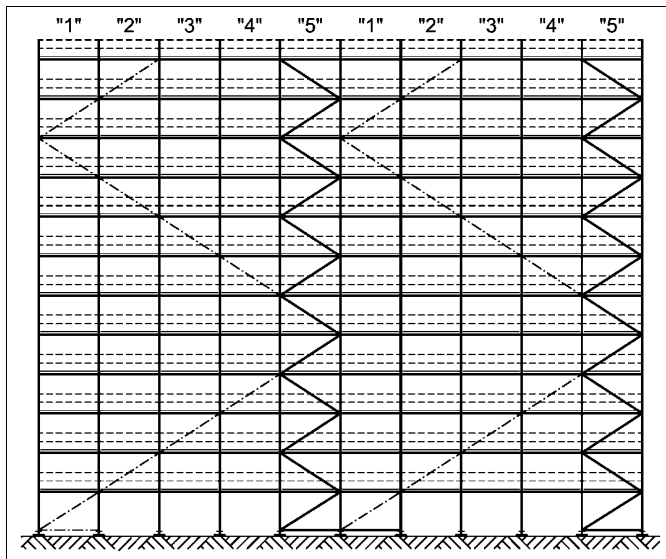
Bild 10: Anordnung der Vertikaldiagonalen
