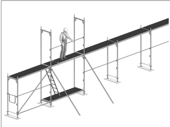
Bild 16: Vorübergehende Kippsicherung der 1. Gerüstlage
