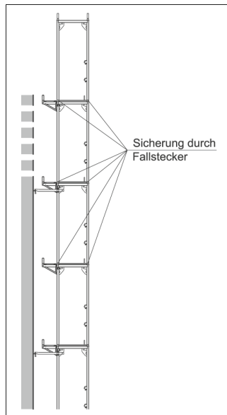
Bild 43: Freistehende Gerüstlagen
