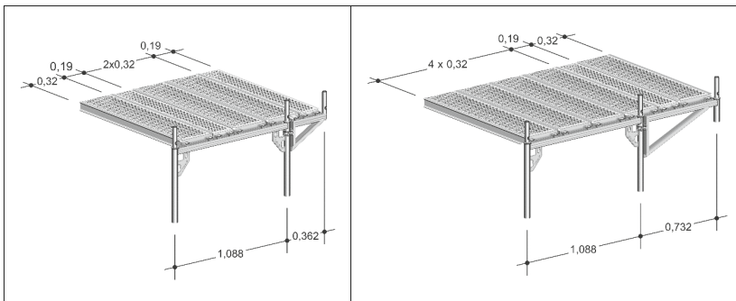
Bild 53: Beispiel zur Anordnung der Böden
