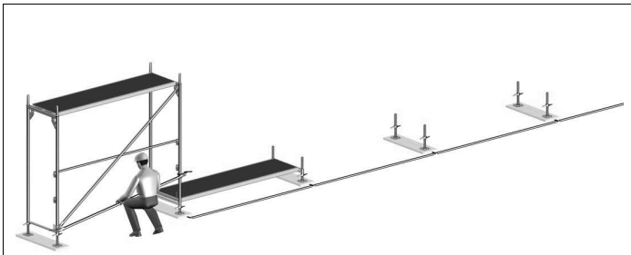
Bild 7: Stellrahmen im Aussteifungsfeld
