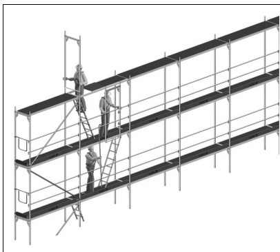
Bild 34: 1. Stellrahmen
