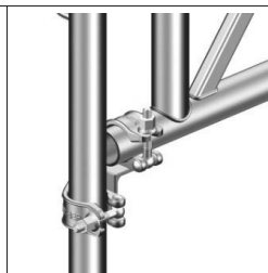
Bild 49: Gitterträgerkupplung
