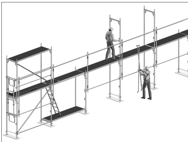
Bild 28: Montage der Gerüstfelder
