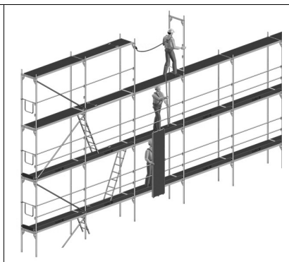
Bild 37: Weitere Gerüstfelder
