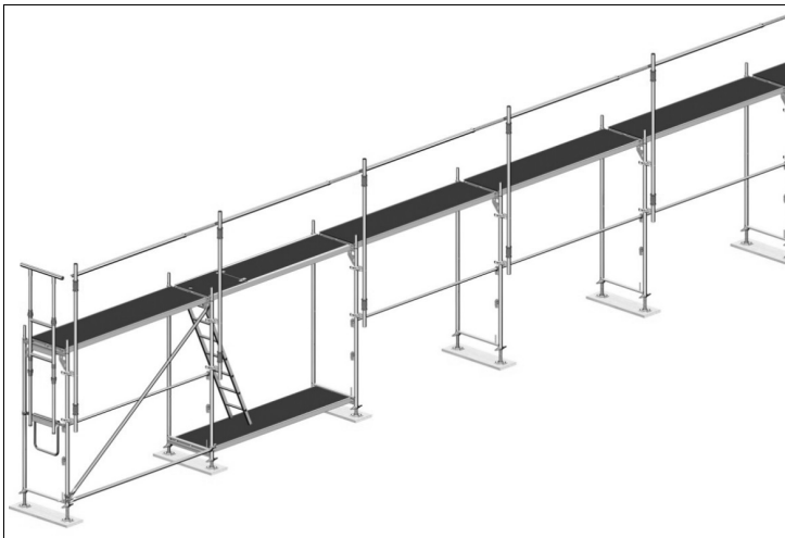
Bild 27: Vorübergehende Sicherung der obersten Lage mit dem MSG
