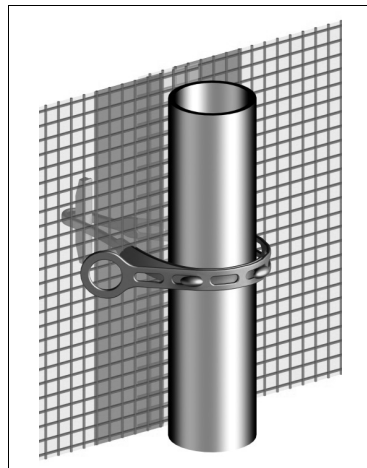
Bild 55: Befestigung von Gerüstplanen (mit Knebelbinder)
