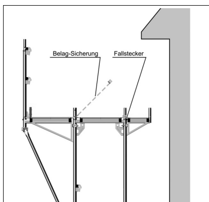
Bild 38: Belagsicherung
