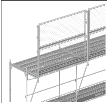
Bild 56: Schutzwand
