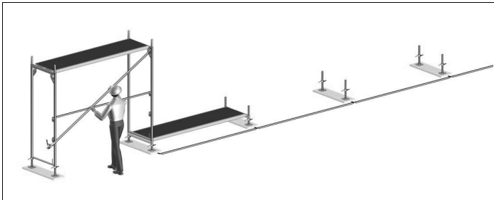
Bild 6: Ausrichten der untersten Gerüstlage
