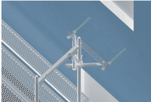
Vertikal versetzter Anker (V-Ankerlösung)
